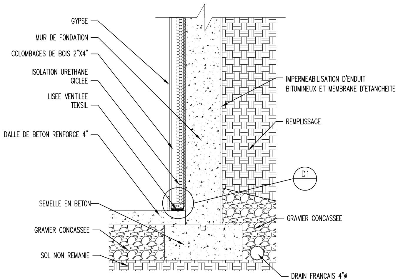
○ APPLICATION TYPIQUE TEKSILL DANS SOUS-SOL ECHELLE: 3/4"=1'-0"
